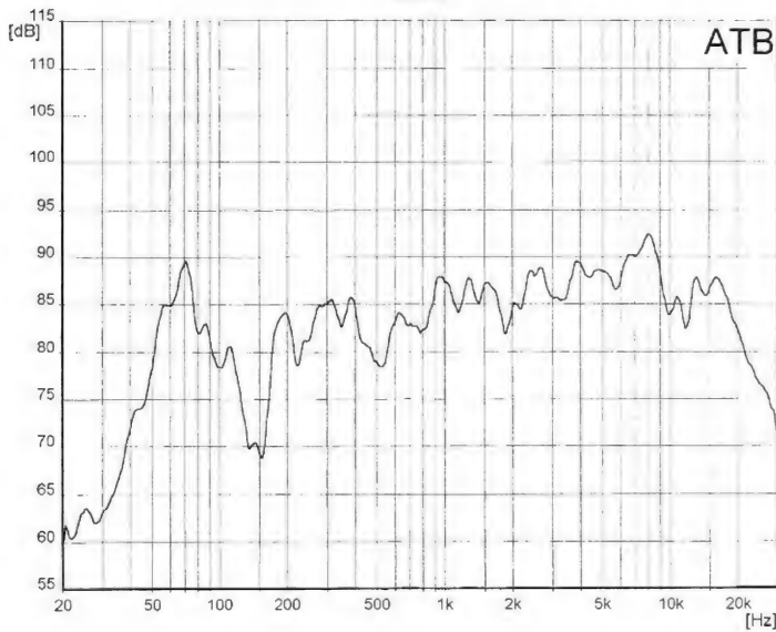
SPL Dimi
